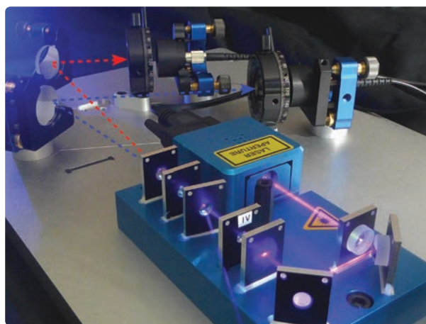
Figur 5 En af de opstillinger man kan arbejde med i QuantumLab. Den intense pumpe laser ( \lambda_p = 405 nm) pumper to ikke-lineære krystaller og via spontan parametriske nedkonvertering (SPDC) konverteres en pumpefoton til et entangled fotonpar ( \lambda = 810 nm) repræsenteret ved de stiplede pile. Fotonerne udbreder sig i to forskellige rumlige retninger; reflekteres igennem individuelle polarisatorer og kobles derefter ind i optiske fibre. Gennem fibre kobles fotonerne til enkeltfotondetektorer og antallet af fotoner der detekteres inden for et koindensinterval på \tau = 25 ns registreres. Foto: Ulrich Hoff.
